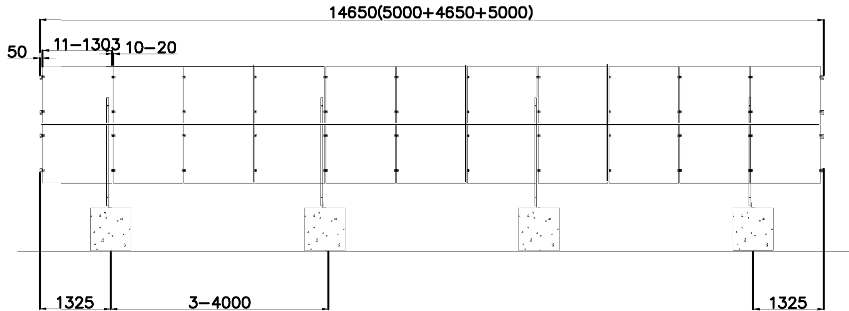
PV Module Layout
